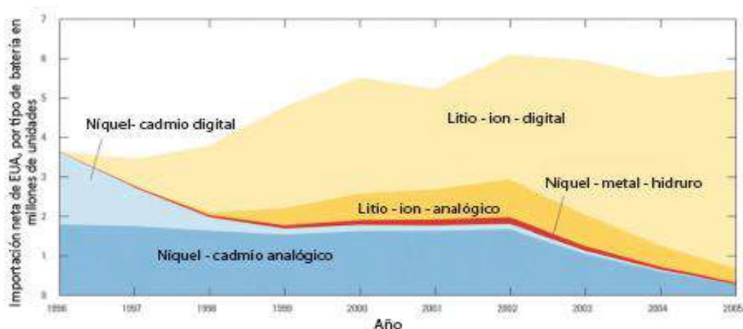
Gráfico N° 2. Importación neta de cámaras de video por tipo de batería (en millones de unidades) (1996-2005).
